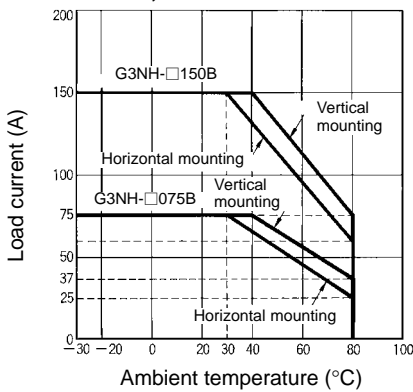
G3NH-□075B, G3NH-□150B
