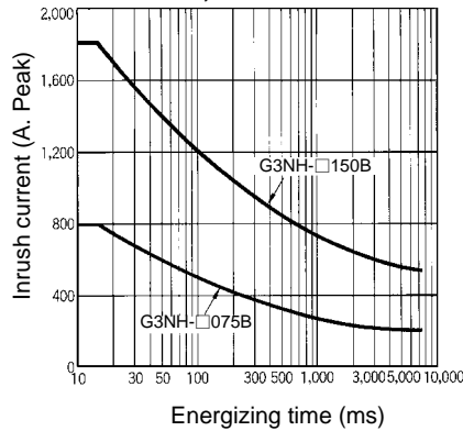
G3NH-□075B, G3NH-□150B
